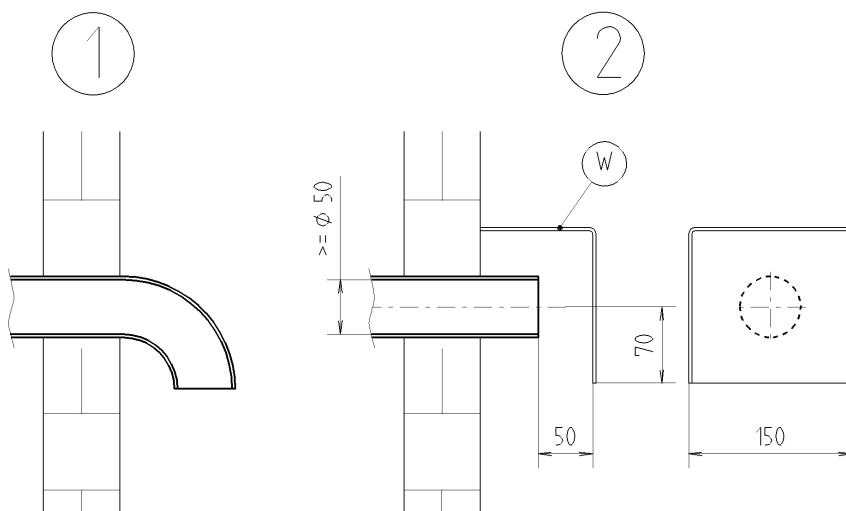
Abbildung 3: Windschutz von Zulufteleitung
